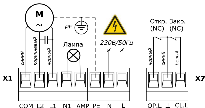
Рис. 6. Электрические подключения привода к модулю управления
