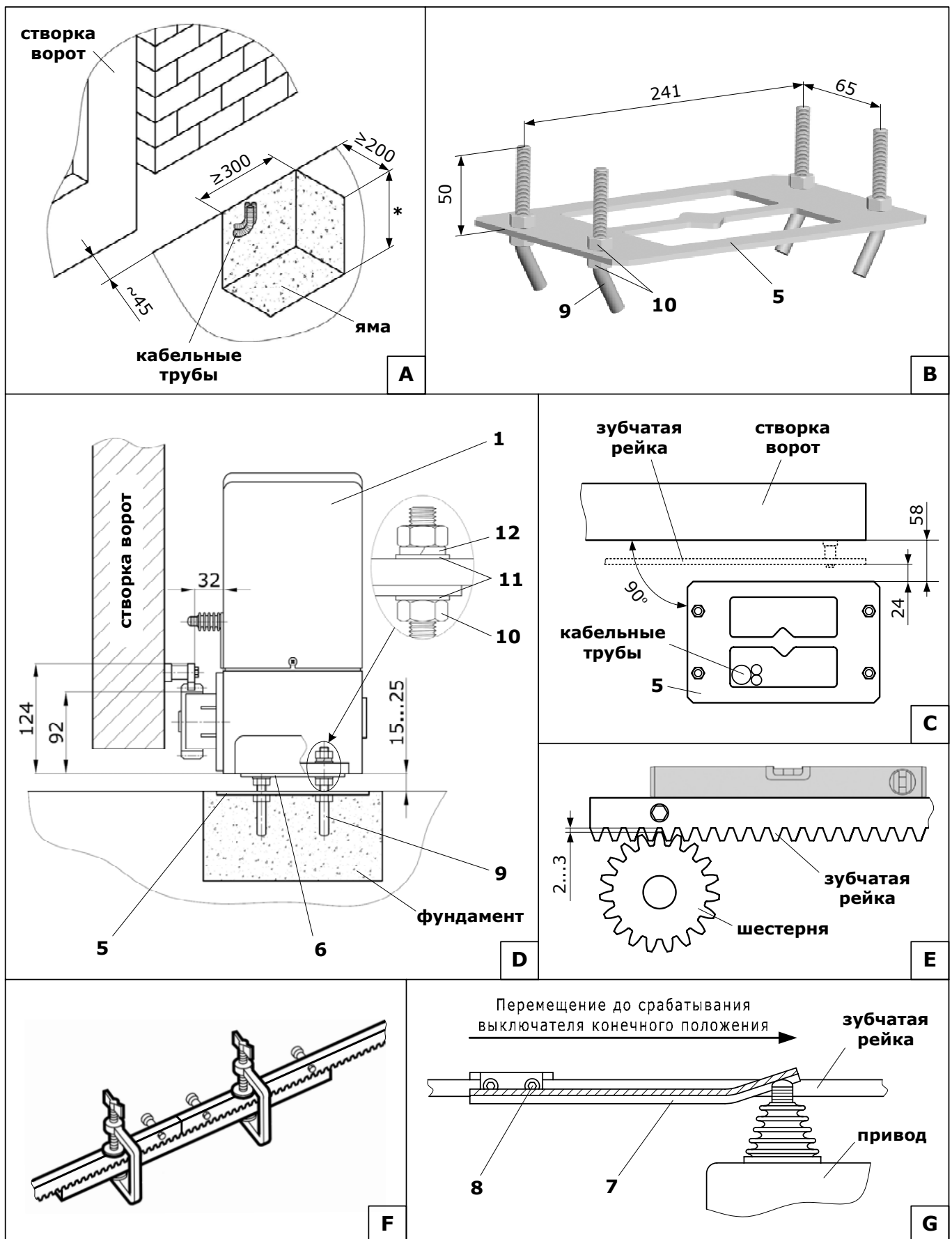
Рис. 3. Монтаж привода
