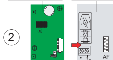
Подключения устройств выполняются только к ВЕДУЩЕМУ приводу
