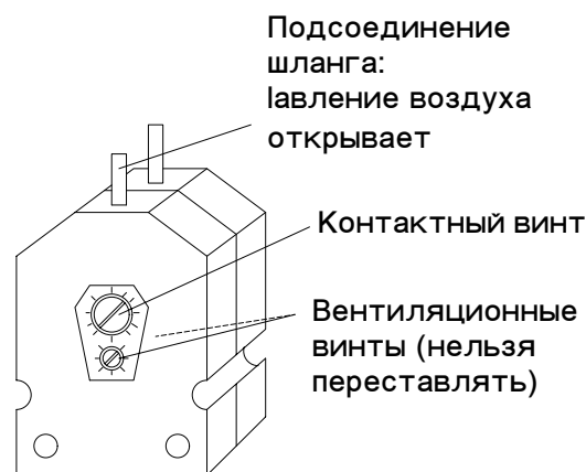
Выключатель давления
